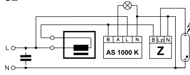
Пусковой переключатель для HS и НИ ламп
