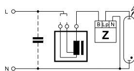
ИЗУ для HS и НИ ламп (ПРА с двумя альтернативными отводами напряжения)
