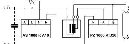
Пусковой переключатель для HS и НИ ламп
