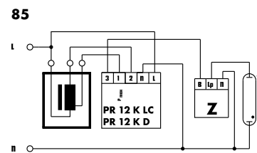
Электронное снижение мощности без фазы управления
