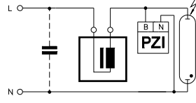
БЗУ для НИ ламп, напряжением зажигания 0,9 кВ
