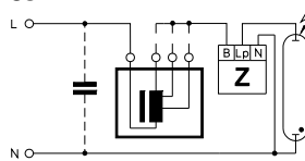
ИЗУ для HS и НИ ламп с тремя альтернативными отводами напряжения
