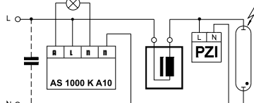
Пусковой переключатель для НИ ламп, напряжением зажигания 0,9 кВ
