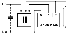
БЗУ HS и НИ ламп
