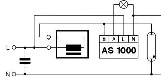
Пусковой переключатель для НМ ламп с вспомогательной лампой
