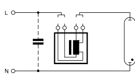
НМ лампы (ПРА с двумя альтернативными отводами мощности и напряжения)
