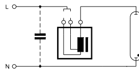
НМ лампы (ПРА с двумя альтернативными отводами напряжения)
