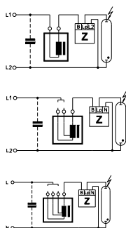
Для Short-Arc ламп
