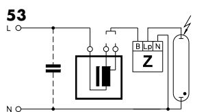
Überlagerungszündung von HS- und HI-Lampen (VG mit zwei alternativen Leistungsanzapfungen)
