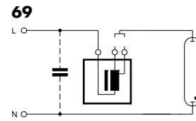
69 HMLampen (VG mit zwei alternativen Leistungsanzapfungen)
