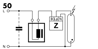
Überlagerungszündung von HS- und HI-Lampen
