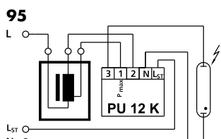
95 Bei zugeschalteter Steuerphase (L ST = 230 V) mit Vorschaltgeräten in zwei Leistungsstufen
