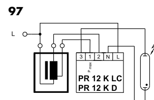
97 Elektronische Leistungsumschaltung ohne Steuerphase
