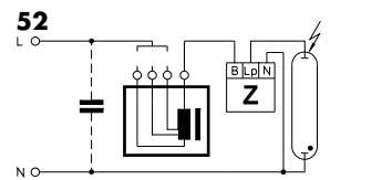
Überlagerungszündung von HS- und HI-Lampen (VG mit drei alternativen Spannungsanzapfungen)
