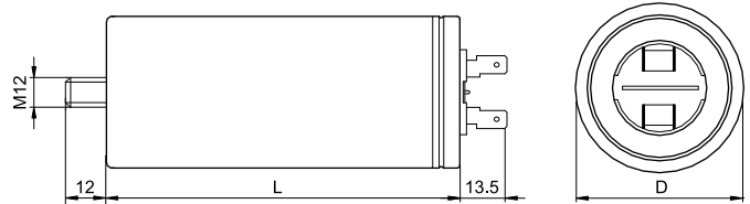
B Doppel-Flachstecker 6,3x0,8 nach IEC 61210
