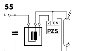
Pulserzündung von Standard-HS-Lampen
