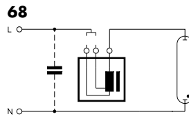
68 HMLampen (VG mit zwei alternativen Spannungsanzapfungen)
