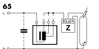
Überlagerungszündung von HS- und HI-Lampen mit drei alternativen Leistungsanzapfungen
