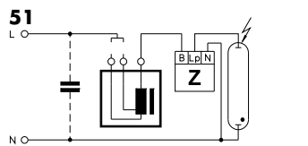
Überlagerungszündung von HS- und HI-Lampen (VG mit zwei alternativen Spannungsanzapfungen)
