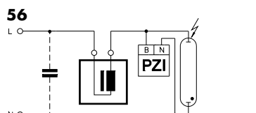
Pulserzündung von HI-Lampen, Zündspannung 0,9 kV
