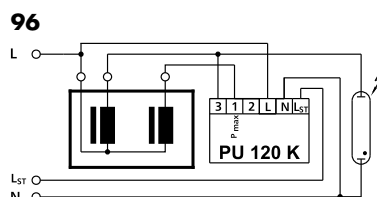
96 Bei abgeschalteter Steuerphase (L ST = 0 V) mit 2 Vorschaltgeräten in Parallelschaltung
