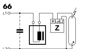
Überlagerungszündung von HS- und HI-Lampen bei Mehrphasennetz
