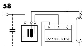
Pulserzündung für HS- und HI-Lampen
