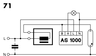
71 Anlaufschalter für HMLampen mit Hilfslampe
